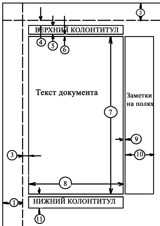
Рис. 1. Параметры страницы
